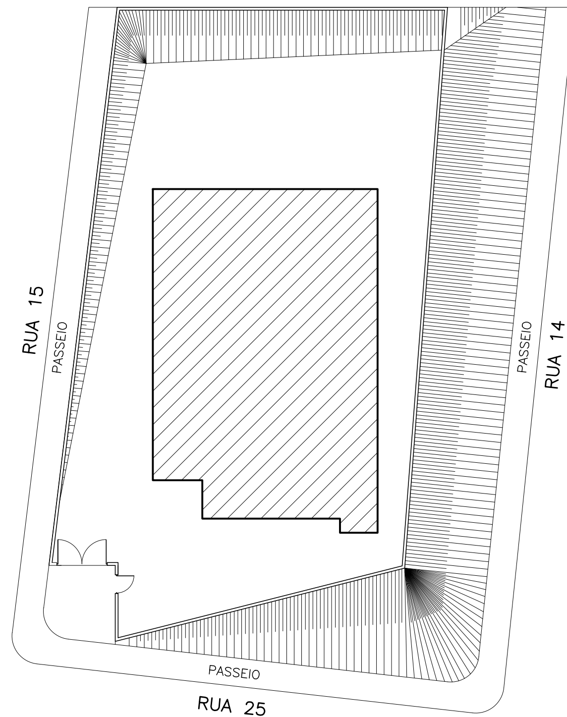
PLANTA DE SITUAÇÃO ESCALA 1:200
