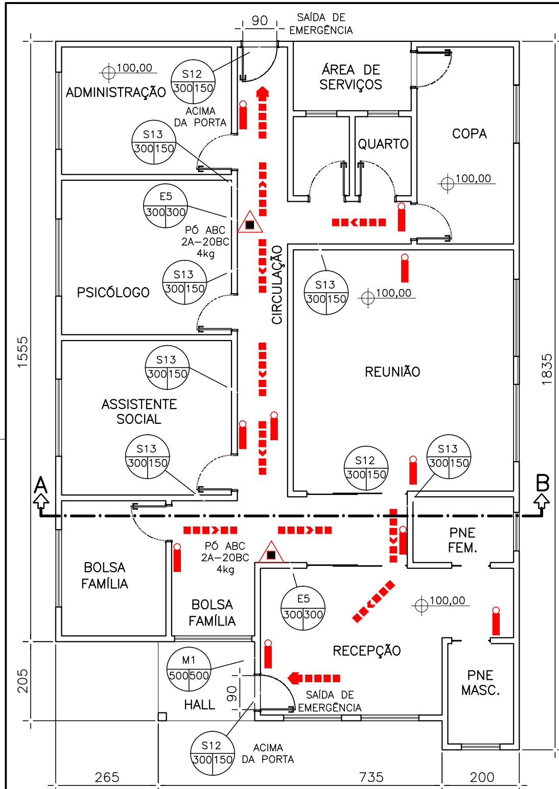
PLANTA BAIXA – TÉRREO ÁREA 207,20m 2 ESCALA 1:100
